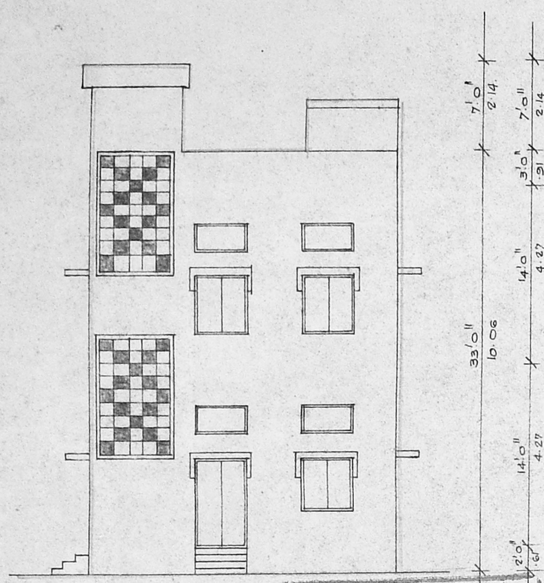
elevation
