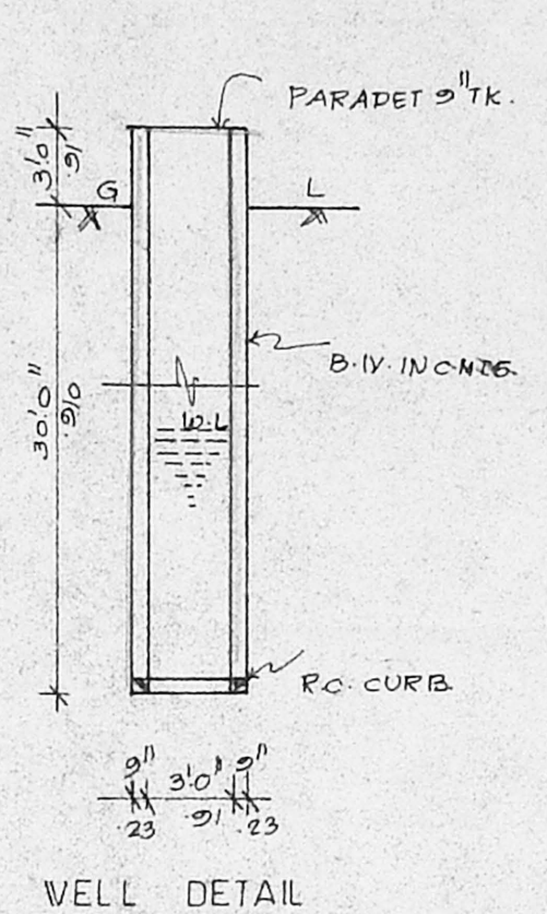
ELEVATION
